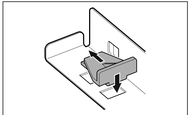
Fig. 53 Anschlagwinkel einsetzen
