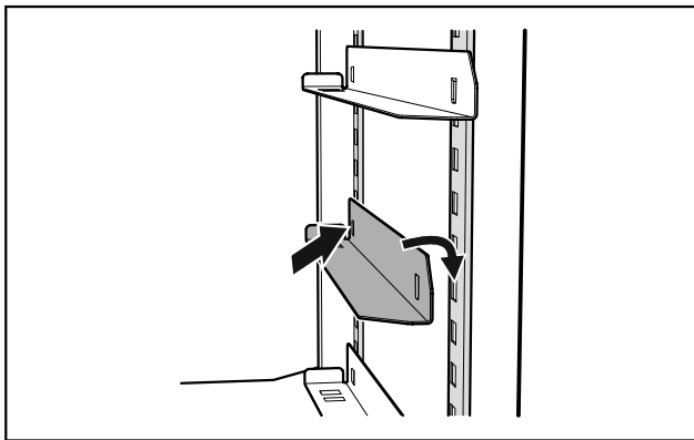
Fig. 51 Auflageschienen
