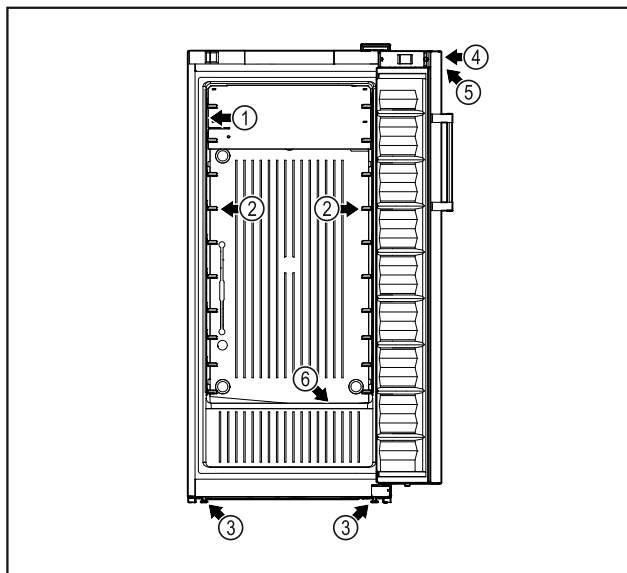
Fig. 1 Beispielhafte Darstellung
