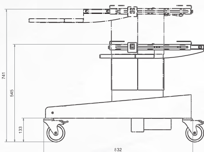
M 50 Fahrgestell elektrisch höhenverstellbar
