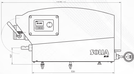
M 50 Antriebsmaschine
