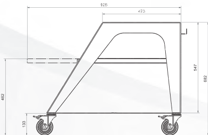
M 50 Fahrgestell
