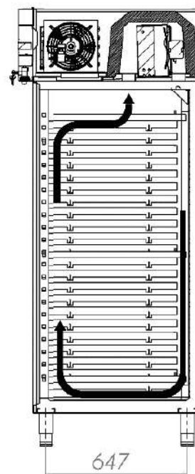
SECTION A-A
