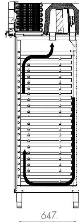
SECTION A-A
